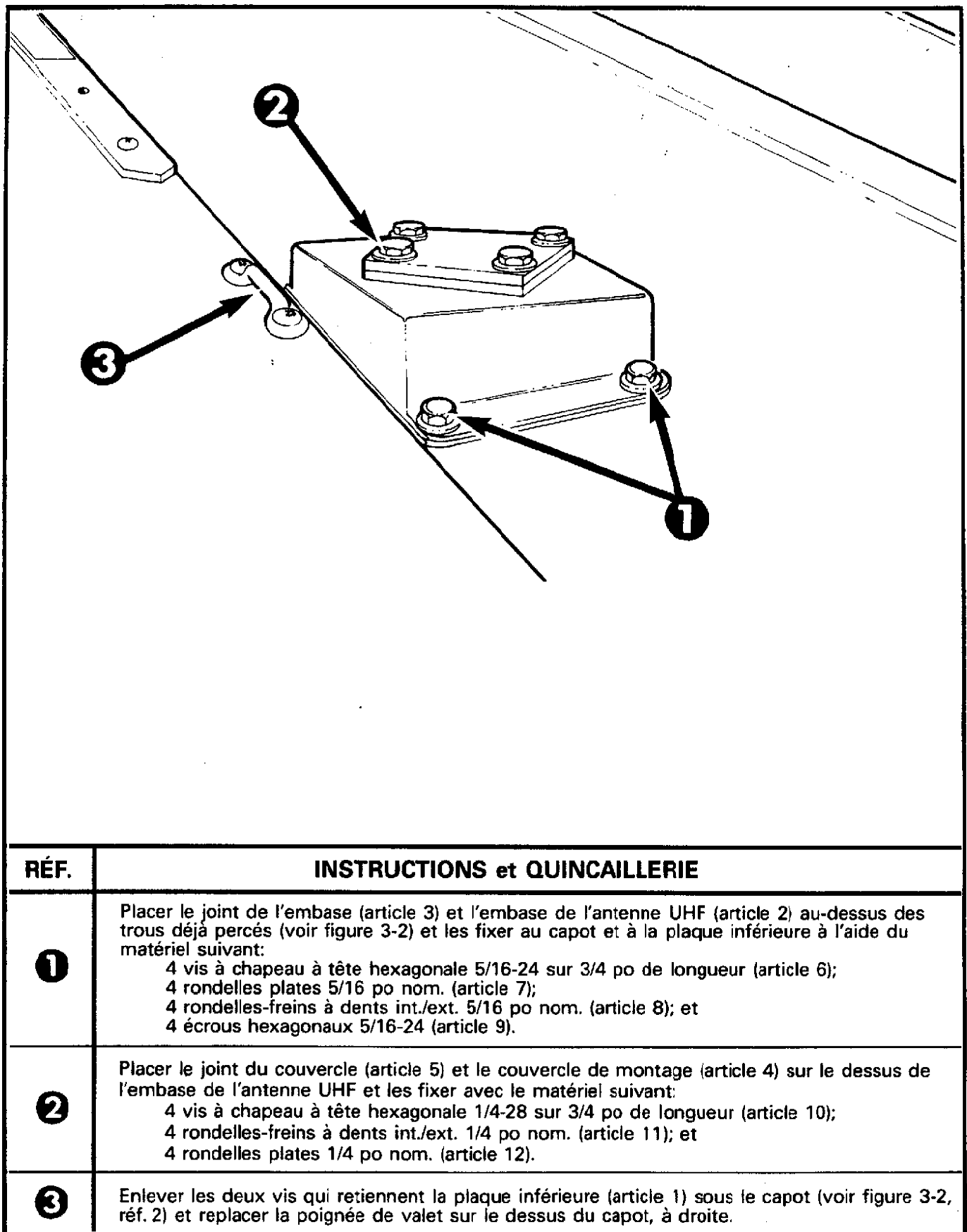
Figure 3-3 Fixation de l'embase d'antenne AT-803/VR
